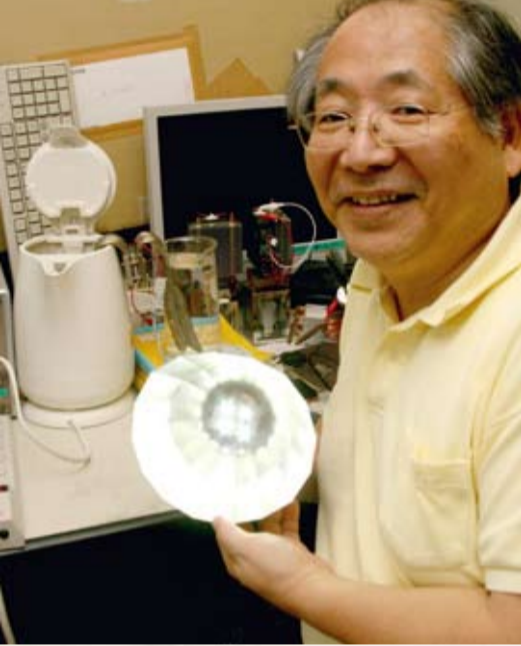
温度差発電実験装置。温泉に見立てボットの熱湯と冷水の入ったヒーターに熱電素子のそれぞれ一端を入れ、その温度差で発電
